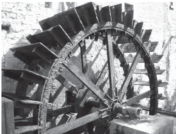
Roue à aubes du Moulin de Fallais
